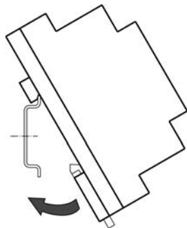
Рис. 5.3. Монтаж прибора с креплением на DIN-реечку
