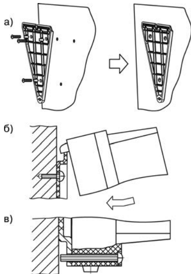
Рис 5.1. Монтаж прибора настенного крепления
