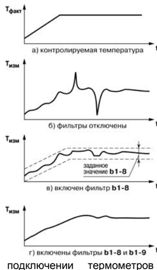
Рисунок 3.2 – Временные диаграммы работы цифровых фильтров
