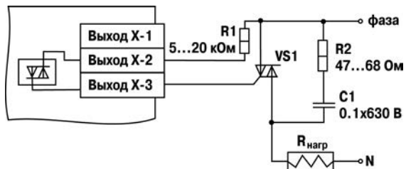
Рисунок Б.3 – Схема подключения силового симистора к ВУ типа С
