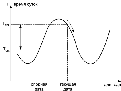
Рисунок 6.2 – График коррекции включения и выключения по восходу и заходу солнца
