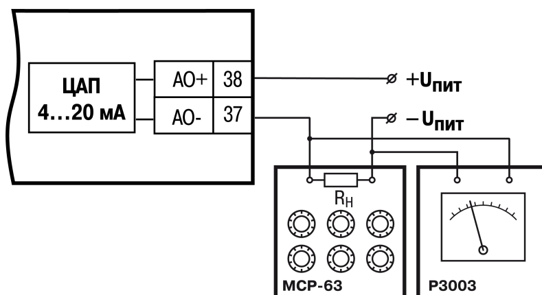
Рисунок 8.4 – Схема подключения к ВЭ типа «И» ( R_H = 500 \text{ Ом} )
