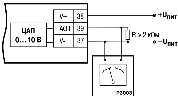
Рисунок 8.6 – Схема подключения нагрузки к ВЭ типа У
