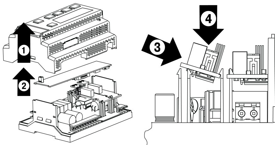
Рисунок 8.13 – Последовательность установки интерфейсной платы
