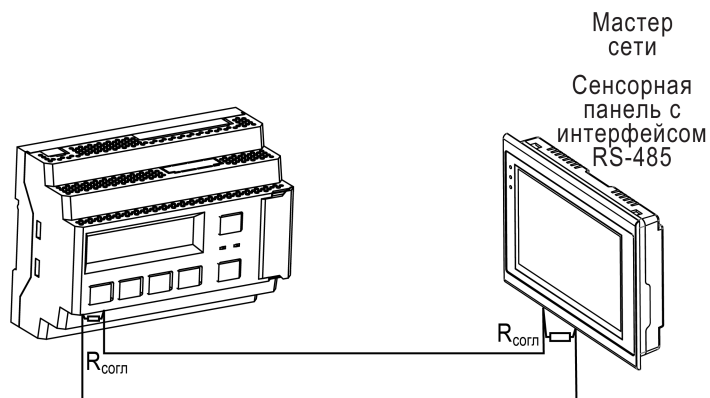
Рисунок 5.16 – Типовая схема подключения для ПР200 в режиме Slave
