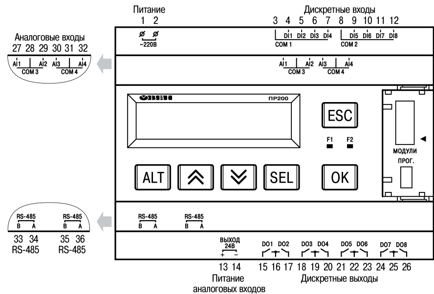
Рисунок А.6 – Расположение контактов ПР200-220.23.2.X
