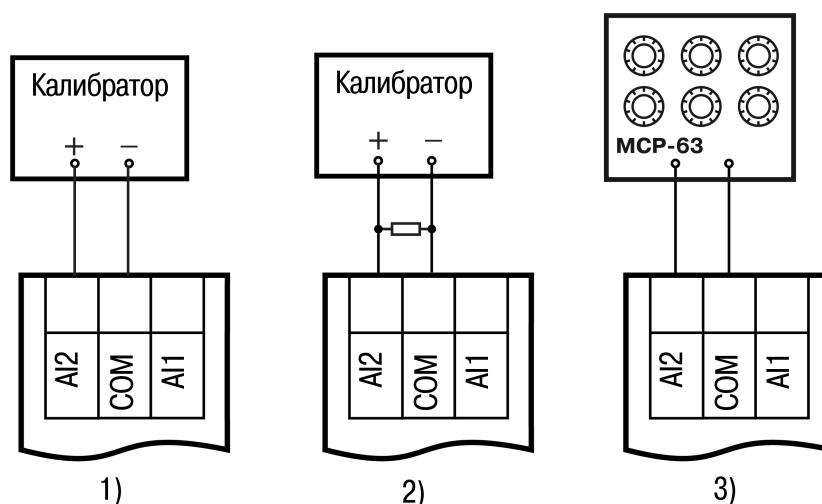
Рисунок 8.1 – Подключение калибратора напряжения
