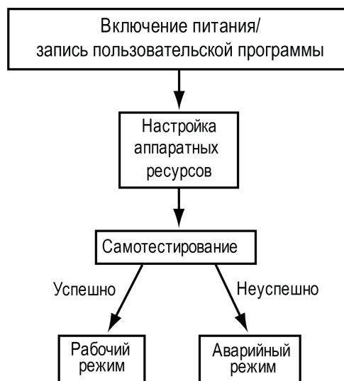
Рисунок 6.7 – Алгоритм запуска прибора
