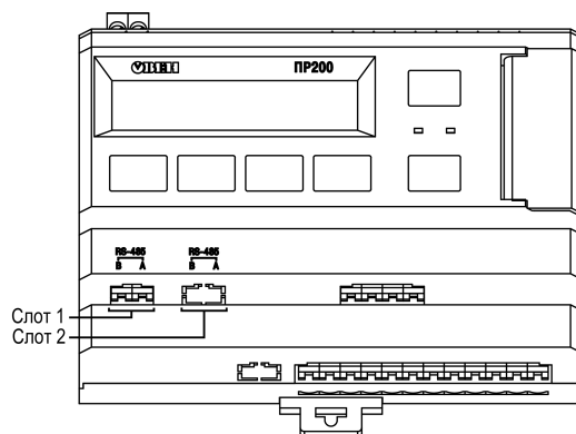
Рисунок 8.12 – Нумерация слотов RS-485
