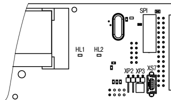
Рисунок 6.9 – Вид на разъем XP3
