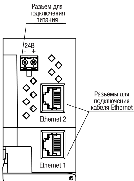
Рисунок 5.2 – Разъемы прибора
