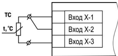
Рисунок Б.2 - Схема подключения термометра сопротивления
