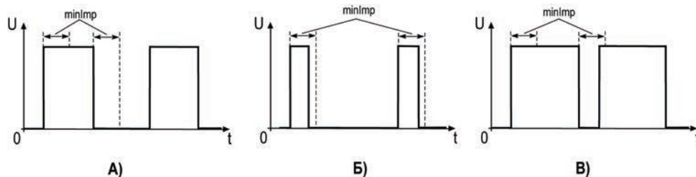
Рисунок 3.2 – Работа параметра minImp
