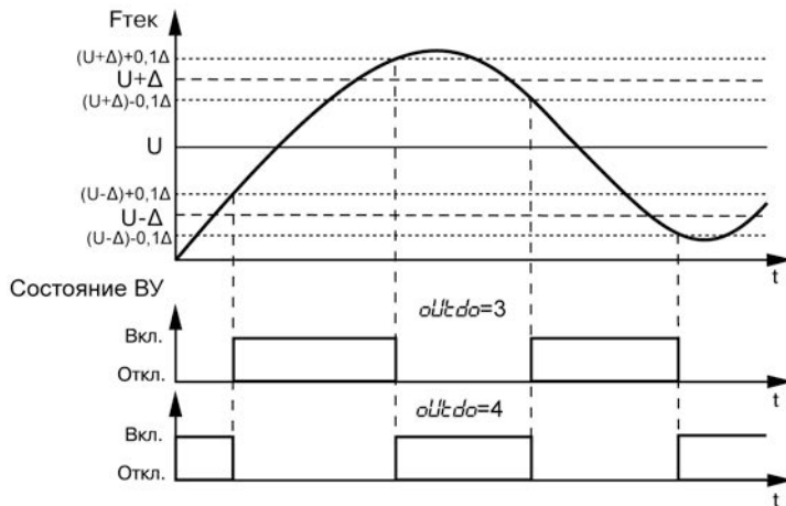
Рисунок 4.2 – П- и U-образная типы логики при работе ВУ в качестве компаратора
