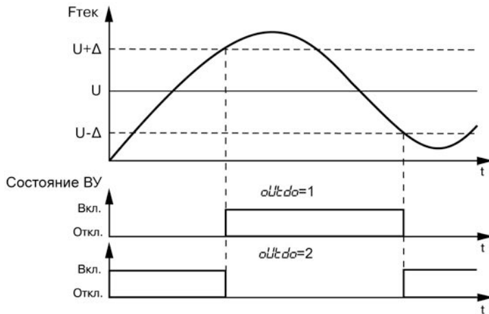
Рисунок 4.1 – Типы логики (обратный и прямой гистерезис) при работе ВУ в качестве компаратора
