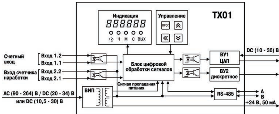
Рисунок 3.1 – Функциональная схема
