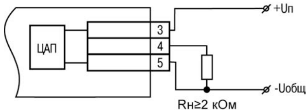
Рисунок Б.5 – Пример подключения ВУ типа У
