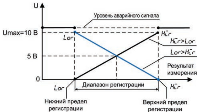
Рисунок 4.6 – Принцип формирования выходного сигнала ВУ в режиме регистратора для приборов с ВУ типа У
