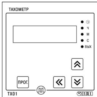
Рисунок 3.3 – Внешний вид лицевой панели прибора для корпуса настенного (Н) крепления
