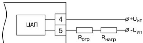
Рисунок Б.4 – Схема соединения ЦАП с нагрузкой для ВУ типа И
