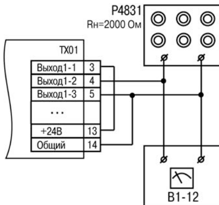
Рисунок Г.1 – Юстировка значений выходного напряжения
