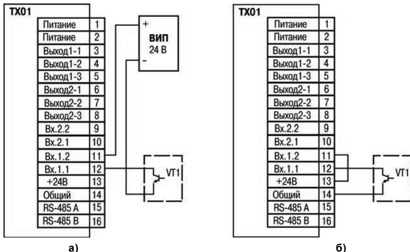
Рисунок Б.1 – Подключение к входу коммутационных устройств: а) при работе датчика от внешнего источника питания; б) при работе датчика от внутреннего источника питания
