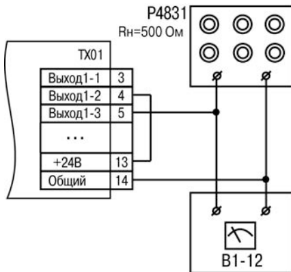
Рисунок Г.2 – Юстировка значений выходного тока
