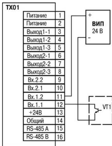
Рисунок Б.2 – Подключение пассивных датчиков, имеющих на выходе транзистор n-p-n типа с открытым коллекторным входом: а) при работе датчика от внешнего источника питания; б) при работе датчика от питающего напряжения прибора
