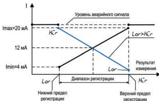
Рисунок 4.5 – Принцип формирования выходного сигнала ВУ в режиме регистратора для приборов с ВУ типа И
