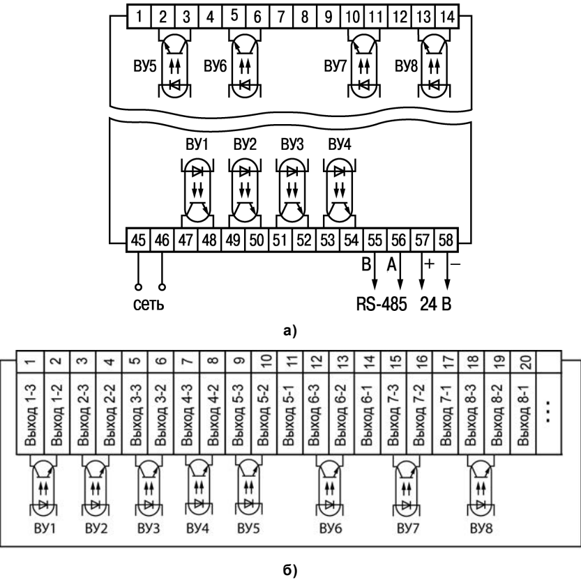
Рисунок Б.3 – Схема подключения транзисторных оптопар прибора ТРМ 138-К: а) в корпусе Щ4, б) в корпусе Щ7
