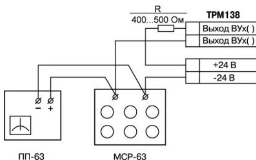
Рисунок Д.6 – Схема подключения аппаратуры при юстировке ЦАП
