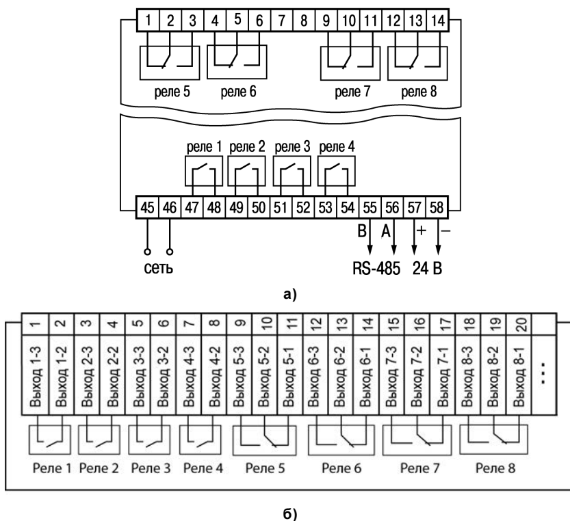
Рисунок Б.2 – Схема подключения электромагнитных реле прибора ТРМ 138-Р: а) в корпусе Щ4, б) в корпусе Щ7
