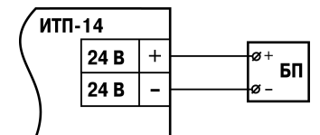
Рисунок 5.1 - Схема подключения к источнику питания
