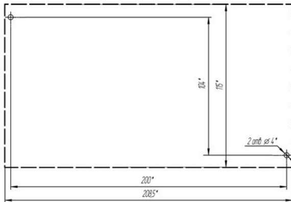
б) ПЛК110.X.60.X-X(M02)
