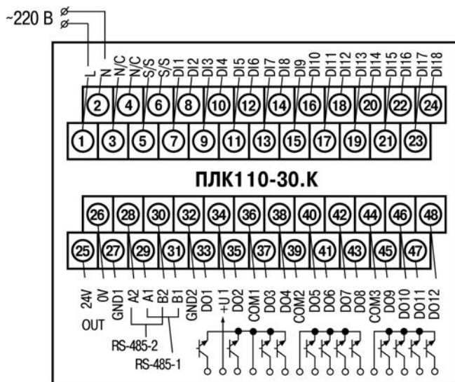
Рисунок Б.6 – Схема расположения и назначение клемм на ПЛК110-220.30.К(М02). Схема для ПЛК110-24.30.К(М02) – аналогична
