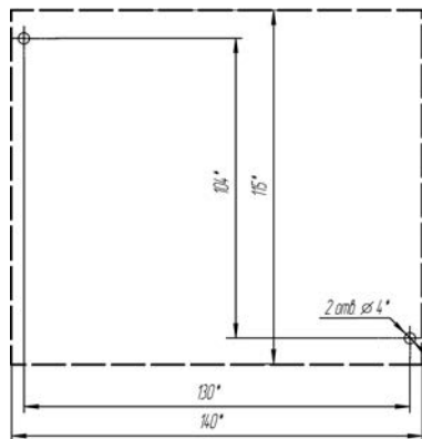
а) ПЛК110.X.30(32).X-X(M02)
