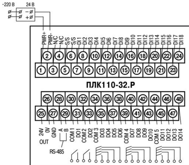
Рисунок Б.3 – Схема расположения и назначение клемм на ПЛК110-24.32.Р(М02). Схема для ПЛК110-220.32.Р(М02) – аналогична
